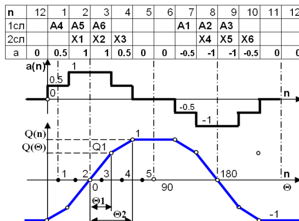
Рис. 1. Построение относительной пространственной обмоточной функции
