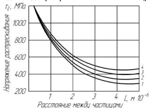
Рис. 3. Напряжения сдвига, необходимые для растрескивания цементитных частиц в стали, в зависимости от расстояния между частицами l ; размеры частиц: 1 – d = 2 мкм; 2 – d = 5 мкм; 3 – d = 10 мкм; 4 – d = 20 мкм
