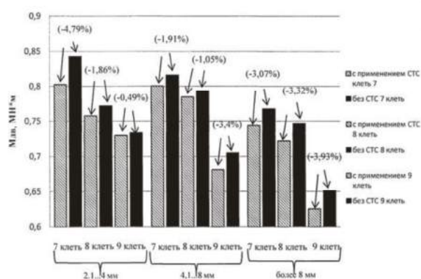
Рис. 2. Усредненное значение M_{пр} в зависимости от толщины прокатываемого металла для 7–9 клеток чистой группы
