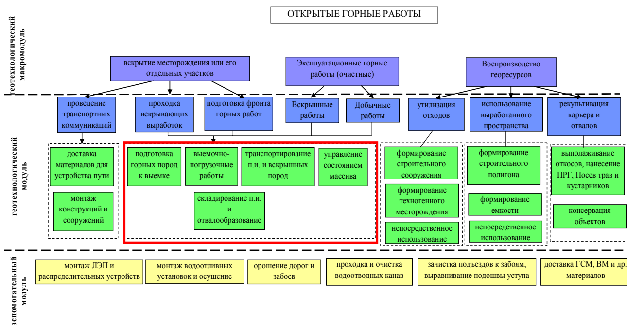
Рис. 1. Структура горнотехнической системы при освоении месторождения открытым способом
