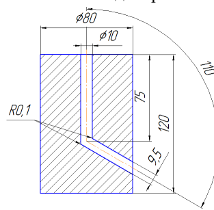
Рис. 1. Форма и размеры матрицы для углового прессования цилиндрических заготовок
