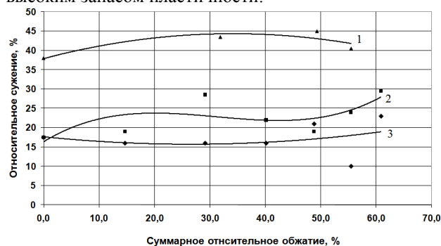
Рис. 4. Зависимость относительного сужения стальных заготовок от их относительного обжатия при волочении: 1- сталь С85CrV; 2, 3 - сталь 85ФЮ
