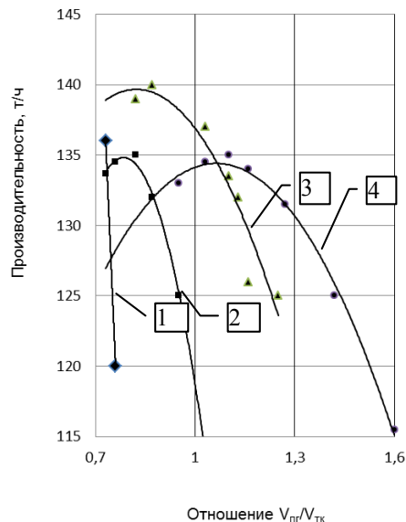
Рис. 1. Зависимость производительности доменной печи от соотношения удельных количеств природного газа V_{\text{пр}} и технологического кислорода V_{\text{тк}} : 1 – 60–79; 2 – 80–99; 3 – 100–119; 4 – 120–140 м³/т чугу.
