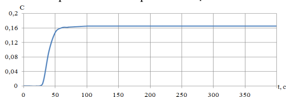
Рис. 3. Графическая зависимость показателя поврежденности c материальной точки от времени
