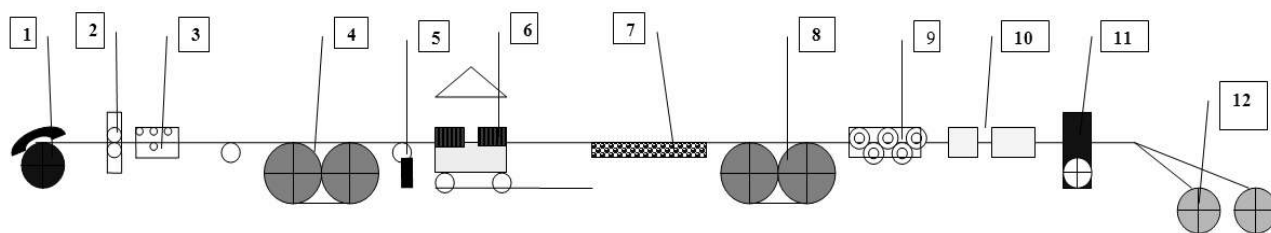
Рис. 1. Схема линии стабилизации арматурной проволоки диаметрами 4–8 мм фирмы «GCR»:
