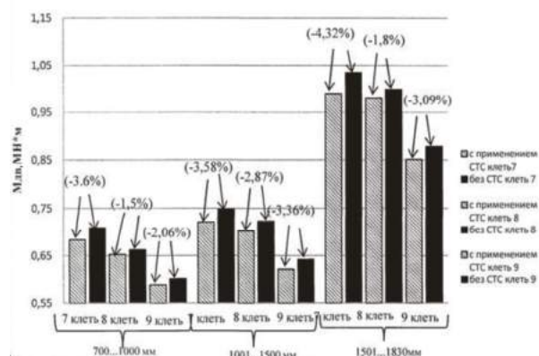
Рис. 3. Усредненное значение M_{пр} 7–9 клеток чистой группы стана 2000 г.п. при различной ширине
