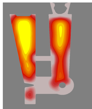
Рис. 5. Влияние соединительных каналов на затвердевание – жидкий металл
