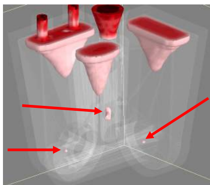
Рис. 11. Усадочная пористость
