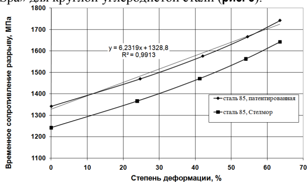
Рис. 3. Изменение временного сопротивления разрыву проволоки из стали 85 на переходах волочения подката, обработанного различными методами (по данным фирм «MFL» и «Continuus Properzi Spa»)
