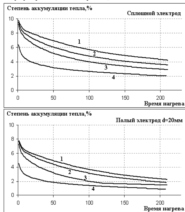
Рис. 1. Динамика изменения степени аккумуляции тепла сплошным и полым электродами. Для всех графиков: 1,2,3,4 – серии из одного, пяти, двадцати и тридцати нагревов соответственно. Время нагрева во всех сериях 3 мин, время между нагревами – 7 мин
