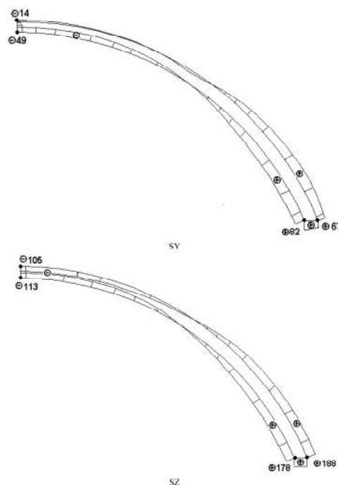
Рис. 4. Эпюры в поперечном сечении, в котором возникают максимальные растягивающие напряжения SY и SZ. Подача 10 мм. Калибровка 105-70-45-140. Угол поворота вала – 118 град
