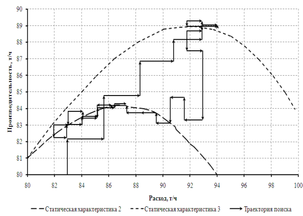
Рис. 4. Расчетные траектории положения статической характеристики G_{\text{вых}}(\tau)=Y(G_{\text{пит}}(\tau)) и траектории изменения G_{\text{вых}}(G_{\text{пит}}(\tau)) в процессе поискового режима: а – при смещении характеристики процесса измельчения при изменении G_{\text{вых}}^{\text{max}} от 70 до 90 т/ч и от 90 до 84 т/ч; б – увеличенное изображение поискового режима работы СОАУ при снижении производительности G_{\text{пит}}^{\text{max}} от 90 до 84 т/ч
