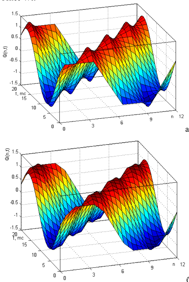
Рис. 3. Пространственно-временные волны МДС двухфазных обмоток \beta=1 (а) и \beta=5/6 (б)
