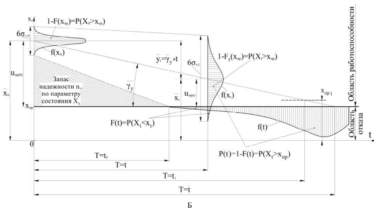
Рис. 2. Графическая интерпретация процесса формирования износных отказов «стационарных» трибосопряжений
