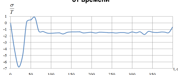
Рис. 6. Графическая зависимость показателя \frac{\sigma}{T} напряженного состояния материальной точки от времени
