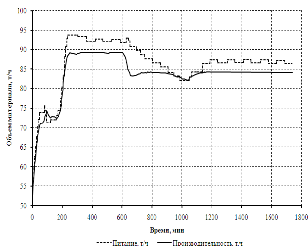
Рис. 3. Траектория изменения во времени G_{\text{пит}}(\tau) и G_{\text{вых}}(\tau) в процессе оптимизирующего режима работы САОУ процессом измельчения при изменении условий, приводящих к смещению статической характеристики процесса измельчения
