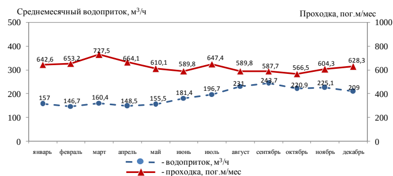
Рис. 2. Динамика среднегомесячного водопритока и среднегомесячной проходки за период 2000–2009 гг. (Шахта «Северная» ОАО «Ургалуголь»)
