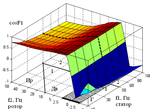
Рис. 1. Зависимость \cos \varphi_1 в функции от частоты питающей сети f_1 и частоты роторной ЭДС f_2
