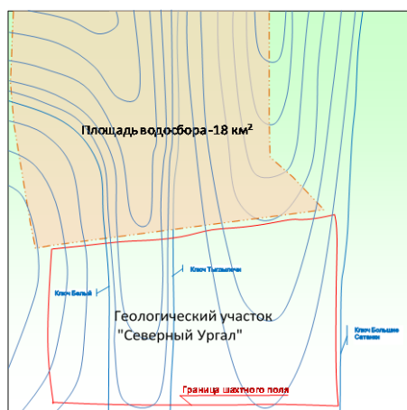
Рис. 5. Схема водосбора поля шахты «Северная» ОАО «Ургалуголь»:
