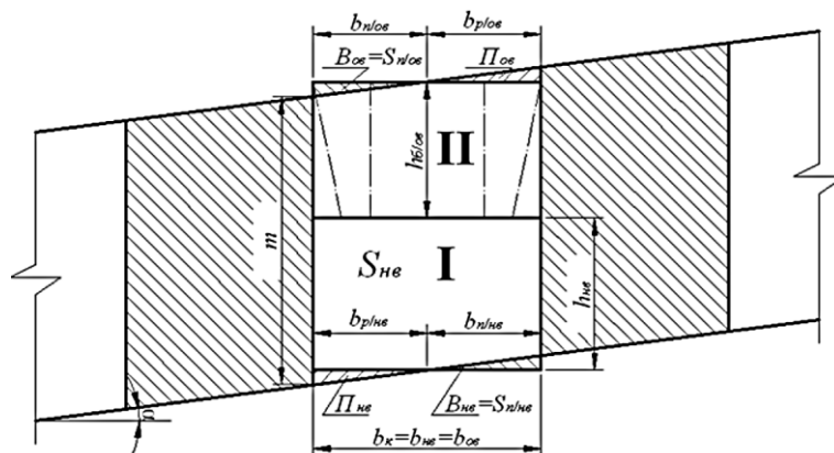
Рис. 4. Схема отработки запасов камеры на руднике «Известняков» с расположением нарезной выработки по почве залежи: I, II – стадии отработки запасов камеры: I – нарезные работы; II – очистные работы; П нв , В нв , П ов , В ов – потери полезного компонента в массиве и подработка вмещающих пород соответственно при отработке нарезной и очистной выработок
