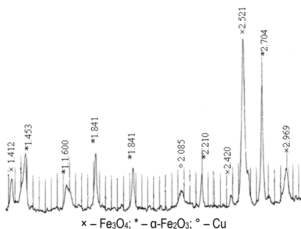
Рис. 2. Рентгенограмма прокаленной смеси оксидного спекa \text{Cu}_2\text{O}-\text{PbO}-2\text{FeO} и \text{Fe}_{\text{мет}} (с поверхности магнитной фракции)
