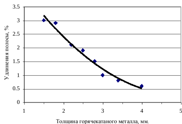
Рис. 2. Удлинение полосы в ИРМ НТА-1 ЛПЦ-5 ОАО «ММК»
