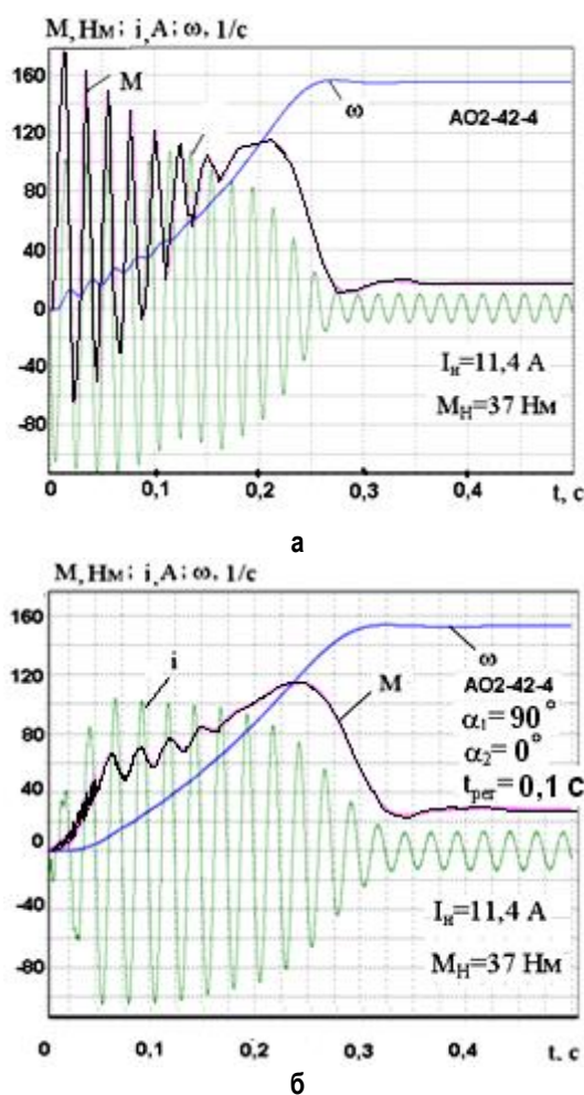
Рис. 3. Расчетные осциллограммы процесса пуска АД при различных условиях
