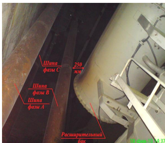
Рис. 1. Монтажное исполнение трансформатора
