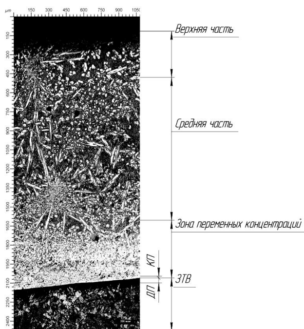
Рис. 1. Панорама строения покрытия 250X15Г20С, \times 100
