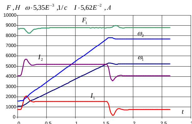
Рис. 9. Переходные процессы в двухконтурной системе с адаптивными регуляторами скорости при пуске стана с заправочной скорости до рабочей
