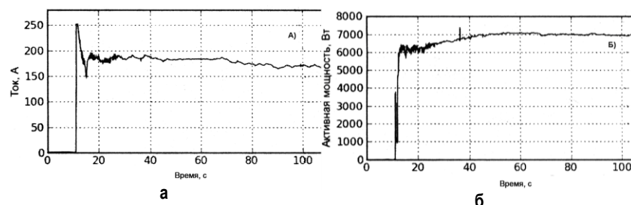
Рис. 5. Процесс поиска оптимального электрического режима электродуговой печи во времени:
