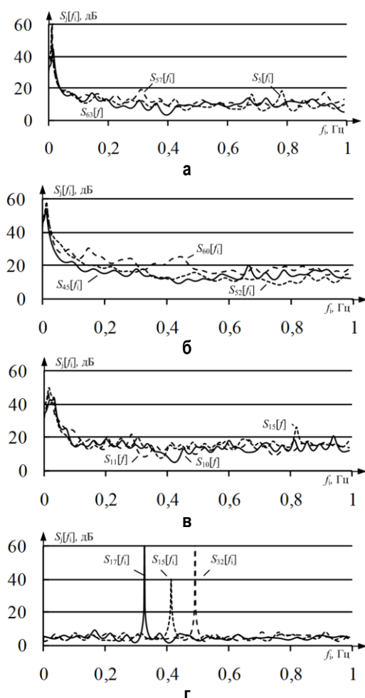
Рис. 1. Графики амплитуд S_i[f] спектральной плотности изменения мгновенных значений моментов нагрузки электродвигателя ТР при прогибе бочки ТР (а), периодической буксовке ТР по слитку (б), износе уплотнительных колец навесного редуктора (в) и износе зубьев шестерней навесного редуктора (г) в интервале частот 0–1 Гц
