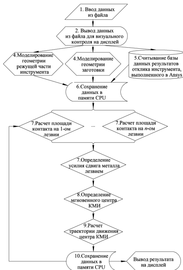
Рис. 6. Блок-схема расчета
