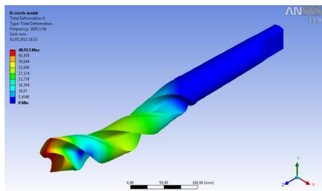
Рис. 5. Пятая форма колебаний
