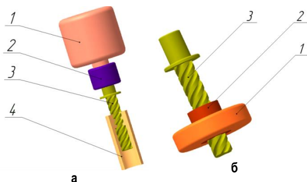
Рис. 2. Винтовые амортизаторы для преобразования амплитудных колебаний в электрическую энергию: а – с генератором на винте: 1 – генератор, 2 – муфта, 3 – винт, 4 – гайка; б – с генератором на гайке: 1 – генератор, 2 – гайка-вал, 3 – винт
