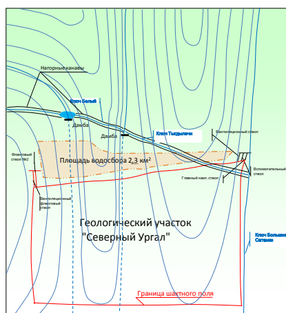
Рис. 5. Схема водосбора поля шахты «Северная» ОАО «Ургалуголь»:
