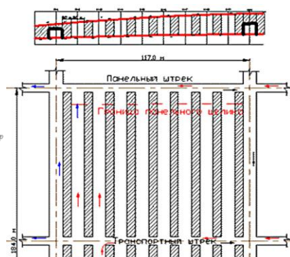
Рис. 3. Камерно-столбовая система разработки на руднике «Известняков»
