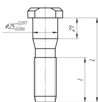
Рис. 1. Колесный болт без рифления
