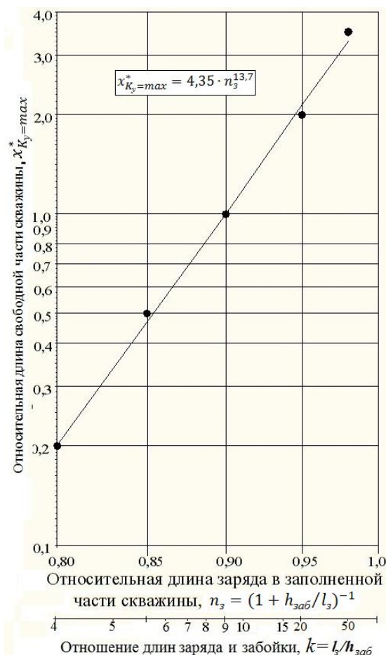
Рис. 4. Зависимость относительных длин заряда и свободной части скважины ( x_{K_y=\max}^* ) при условии достижения K_y^{\max}
