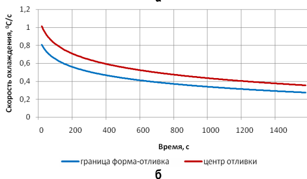
Рис. 2. Скорости охлаждения щелочестойкого состава: а – форма с теплоизолятором – асбест; б – песчано-глинистая форма
