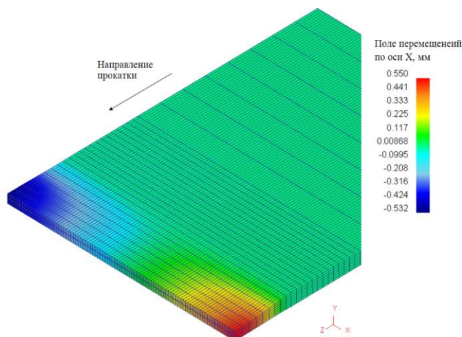
Рис. 4. Поле перемещений в очаге деформации при прокатке ленты с клиновидным поперечным сечением ( \varepsilon=30\% , \mu=0,1 )
