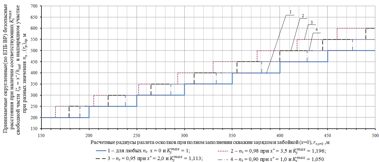
Рис. 6. Принимаемые безопасные расстояния (r_p)_{np} для максимальных увеличений ( K_y^{max} ) зон разлета при разных относительных длинах свободной части ( x^* = l_{св}^* / h_{заб} ) и фиксированных значениях длин заряда в заполненной части n_3 = (1 + h_{заб} / l_3)^{-1} скважин в зависимости от расчетного безопасного расстояния r_{p, x=0; n_3} при заполненной до устья ( x = 0 ) скважине
