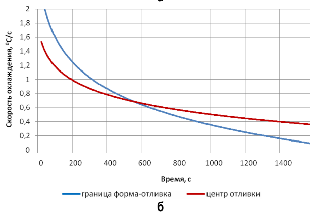
Рис. 4. Скорости охлаждения термостойкого состава: а – форма с теплоизолятором – асбест; б – песчано-глинистая форма
