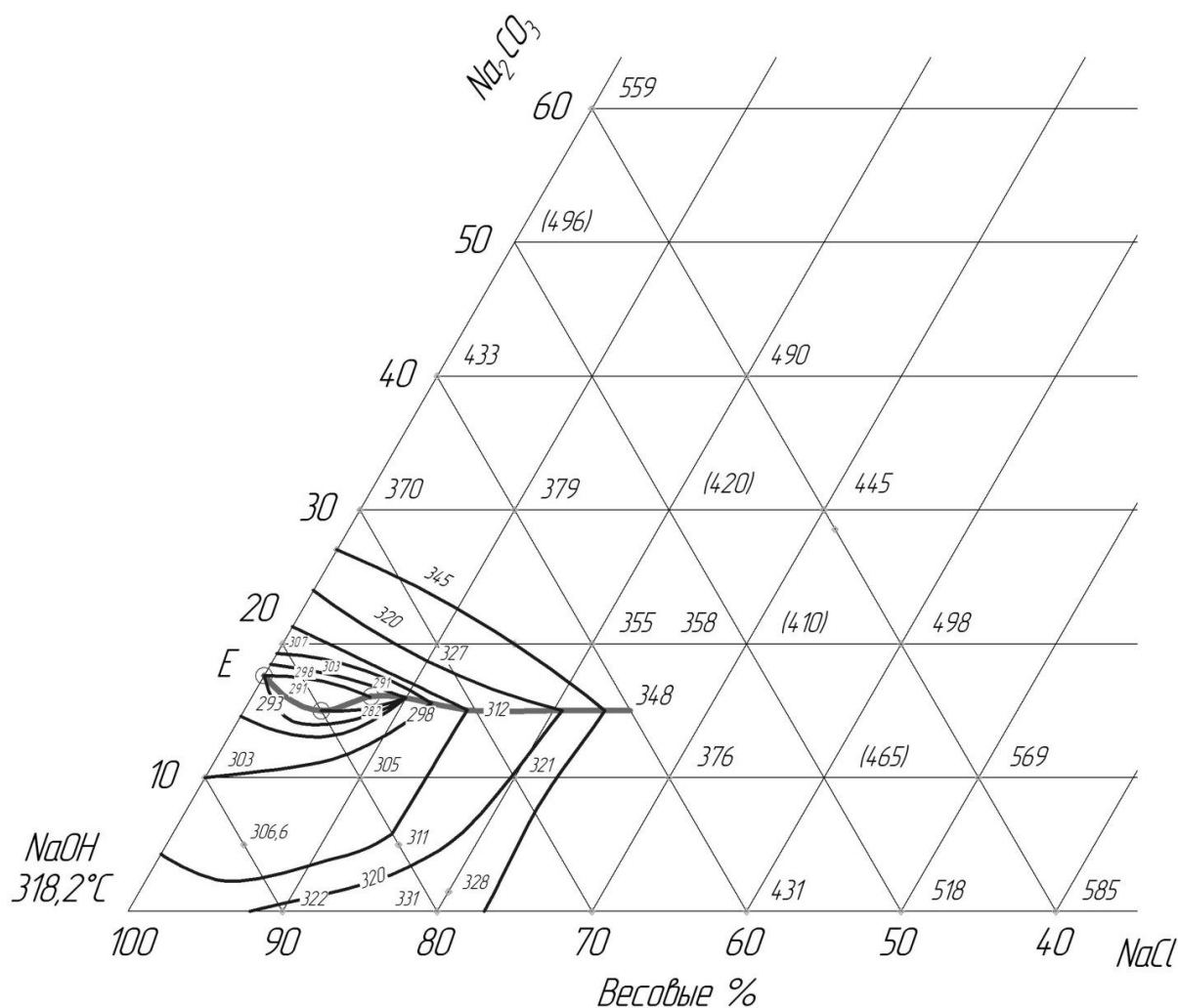
Рис. 1. Диаграмма плавкости системы \text{NaOH}-\text{Na}_2\text{CO}_3-\text{NaCl}
