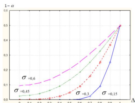
Влияние величин \sigma и \Delta' на долю брака (1 - \alpha)
