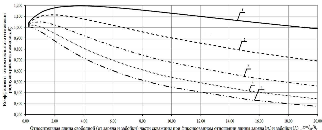
Рис. 2. Коэффициент относительного (по сравнению с целиком заполненной скважиной) изменения радиусов разлета осколков ( K_y = r_{p,x}/r_{p,x=0} ) в зависимости от относительной длины ( x = l_{св}/h_{заб} ) свободной части в надзарядном участке скважины при фиксированных относительных длинах заряда и забойки
