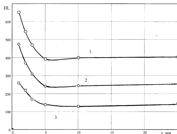
Рис. 8. Изменение условной твердости в зависимости от толщины оболочки радиусом 25 мм: 1 – \sigma_T = 1000 МПа; 2 – \sigma_T = 450 МПа; 3 – \sigma_T = 200 МПа
