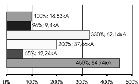
Рис. 2. Характер изменения токов КЗ в сети 110 кВ
