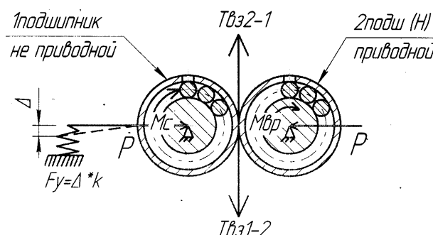
Рис. 1. Схема экспериментальной установки для проведения экспериментов: Твз2-1 и Твз1-2 – силы взаимодействия роликов; Мс – момент сопротивления; Мвр – момент вращения; Δ – величина отклонения тензометрической пластины от исходного положения; Fy – сила упругости тензометрической пластины; k – коэффициент упругости
