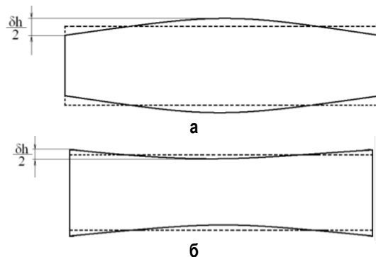
Рис. 9. Форма поперечного сечения ленты: а – выпуклая; б – вогнутая
