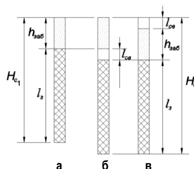
Рис. 1. Элементы конструкции скважинного заряда:
