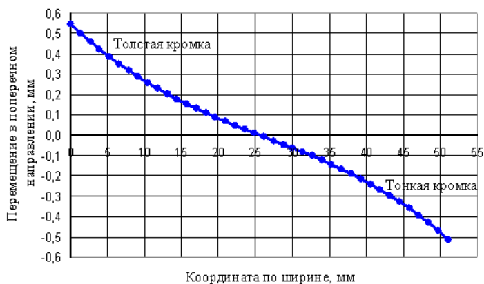
Рис. 5. Перемещение частиц металла в поперечном направлении
