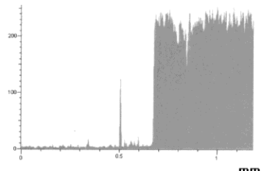
Iron Ka1
