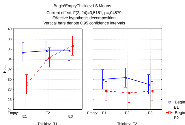
Рис. 2. Эффект взаимодействия фактора толщины металла T со взаимодействием факторов B \cdot E
