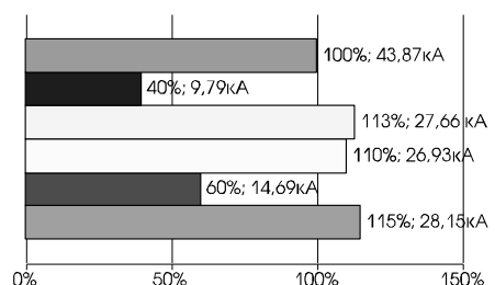
Рис. 3. Характер изменения токов КЗ в сети 220 кВ
