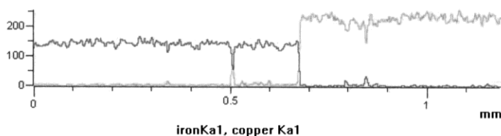
Рис. 5. Спектры медного покрытия и стального сердечника
