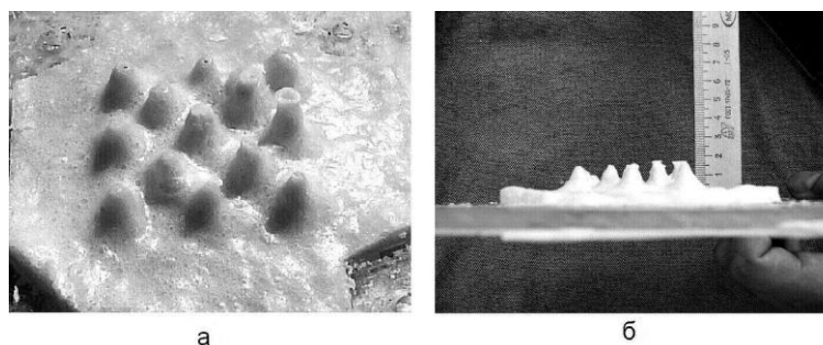
Рис. 5. Образец парафинового гарниссажа, полученный в ходе экспериментов: а – общий вид; б – вид сбоку
