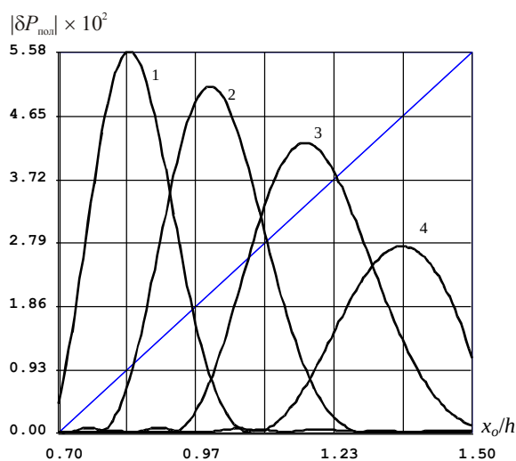
Рис. 2. Зависимость нормированной амплитуды принимаемого сигнала для дефекта типа «полоса» от нормированного расстояния до центра системы преобразователей для различных углов ввода: 1 – \alpha=40^\circ ; 2 – 45^\circ ; 3 – 50^\circ ; 4 – 55^\circ
