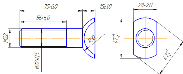
Рис. 1. Болт клеммный по ОСТ 32.161-2000
