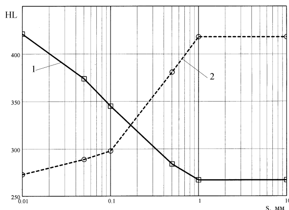
Рис. 15. Изменение условной твердости в зависимости от толщины поверхностного слоя с более низкой (1) и более высокой (2) твердостью, чем основной металл
