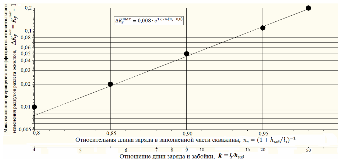
Рис. 3. Максимальное относительное приращение \Delta K_y^{\max} = K_y^{\max} - 1 радиуса разлета осколков в зависимости от относительной длины заряда n_3 = (1 + h_{\text{заб}}/l_3)^{-1} в заполненной части скважины при значениях x^* = l_{\text{св}}^*/h_{\text{заб}} , соответствующих максимуму K_y для заданного n_3
