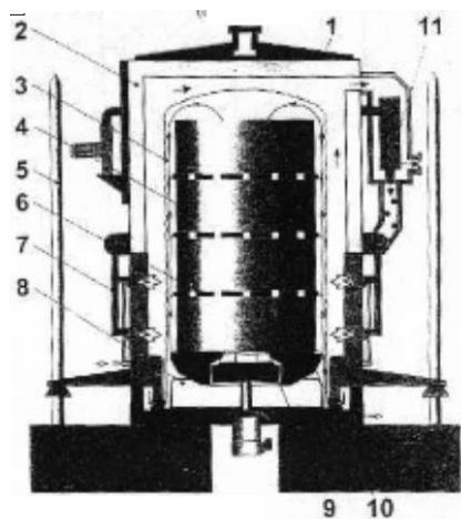
Рис. 1. Схема стенов с нагревательным колпаком:
