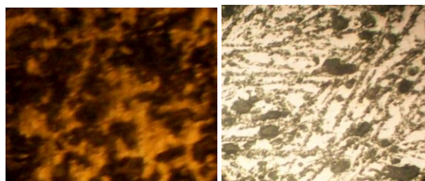
Рис. 5. Структура образцов, закристаллизованных в ПГФ с теплоизолятором, ×500: а – износостойкий; б – кислотостойкий; в – щелочестойкий; г – термостойкий
