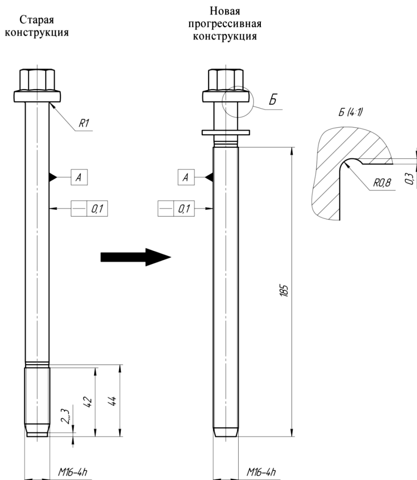
Рис. 5. Конструкции фланцевого болта крепления блока цилиндров
