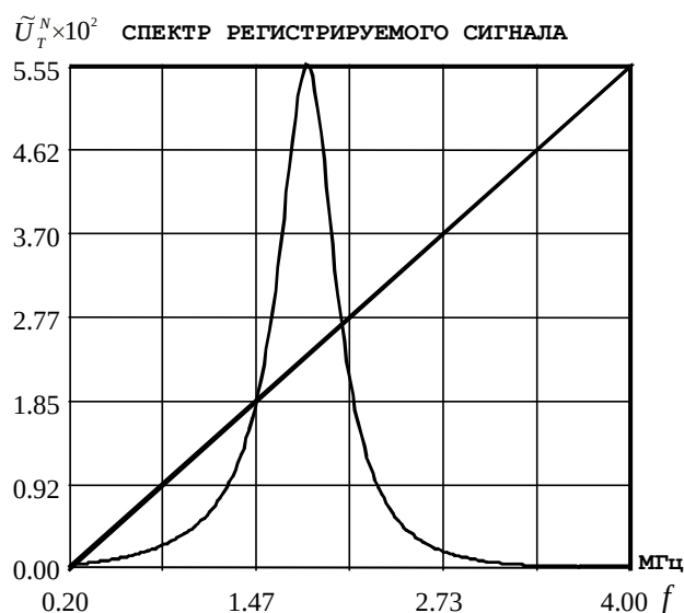
Рис. 6. Теоретический частотный спектр сигнала от отверстия Ø6 в образце СО-2 для преобразователя типа ПЦП-45-КТ в эхоимпульсном режиме
