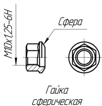
Рис. 4. Сферическая гайка крепления форсунки
