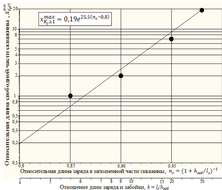
Рис. 5. Зависимость предельных (для K_y \geq 1 ) относительных длин свободной части скважины ( x_{K_y \geq 1}^{max} = l_{св}^* / h_{заб} ) и длины заряда n_3 = (1 + h_3 / l_3)^{-1} в её заполненной части
