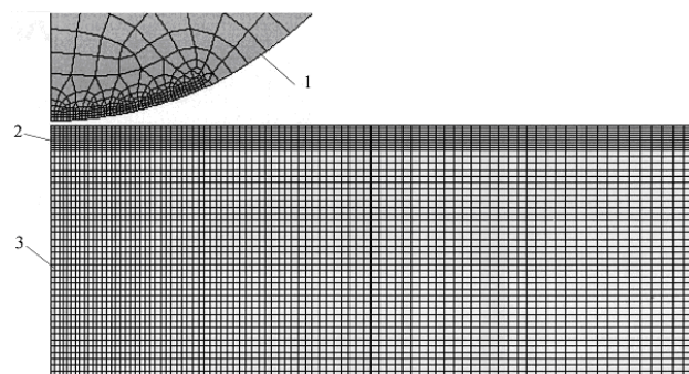
Рис. 14. Конечноэлементная модель удара 1 (показана нижняя часть) и ударяемого тела с различными механическими свойствами по толщине (в слоях 2–3)
