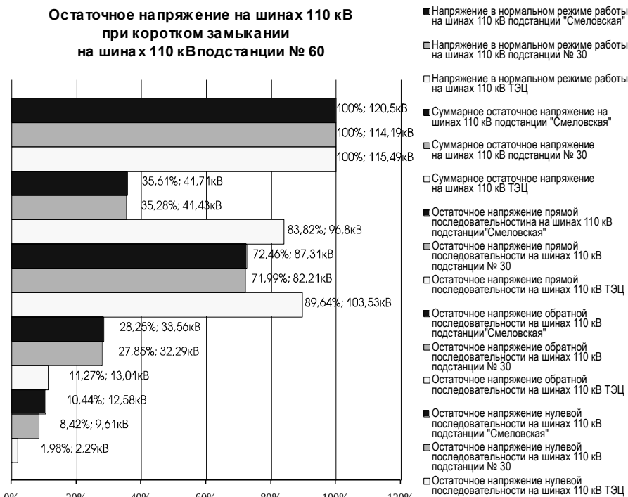
Рис. 5. Уровни остаточных напряжений при КЗ на шинах 110 кВ ПС № 60
